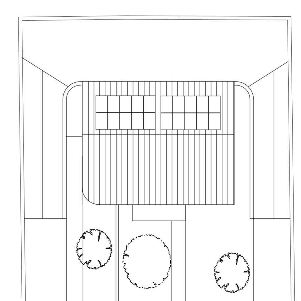
PLANIMETRIA
